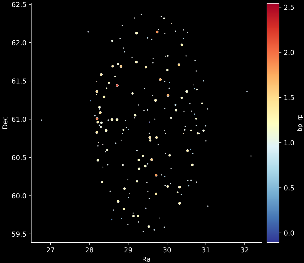
APOGEE DR17 Field: [CVZ_OB17_btx] Stars: 186
