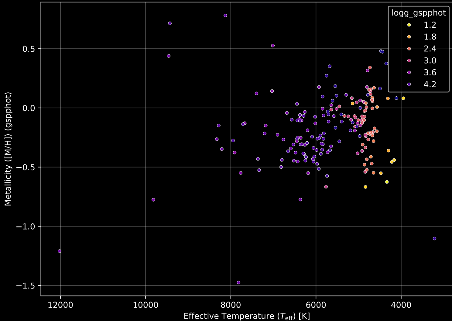
APOGEE DR17 Field: [CVZ_OB17_btx] Stellar Population Parameters (n= 186)
